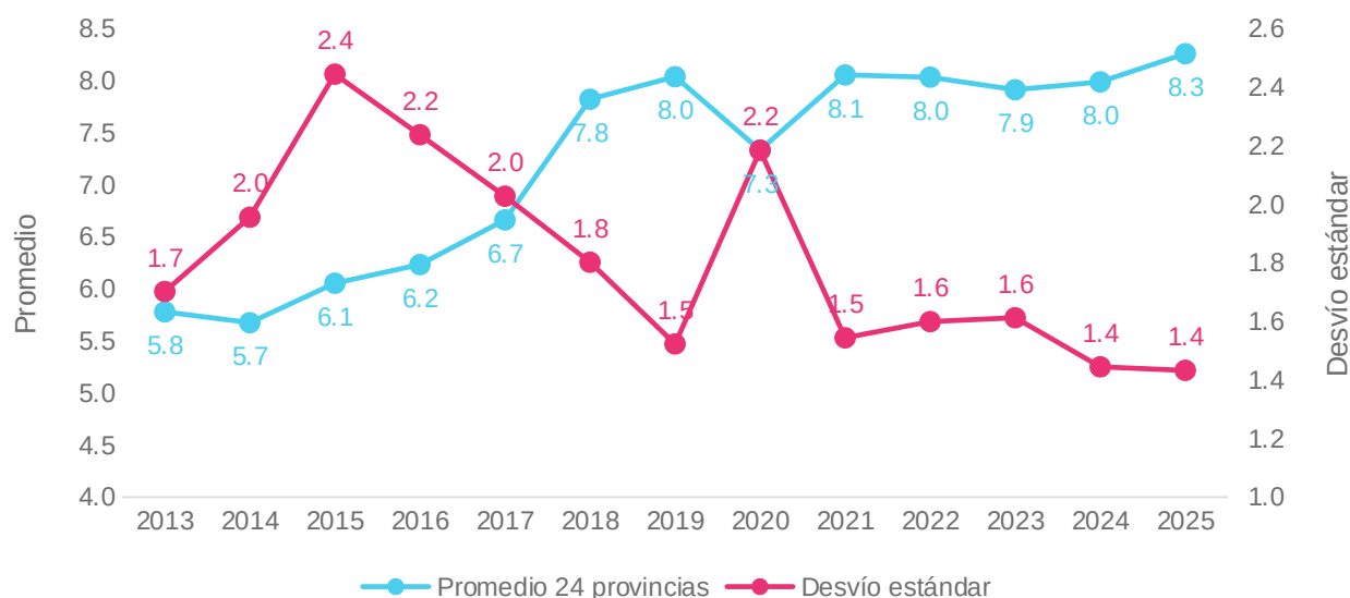
Gráfico 1. Serie de tiempo promedio y desvío estándar
